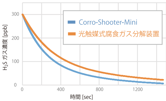
除去ガス: 硫化水素, 試験開始濃度: 300ppb, 試験容積: 0.25m 3
